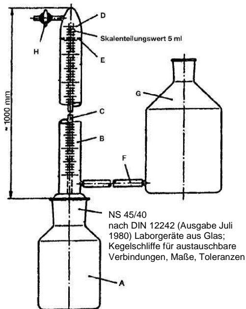
Bild 2: Versuchsanordnung zur Bestimmung des Faulverhaltens von Schlamm nach DIN 38414-8, Seite 6, Ausgabe Juni 1985
