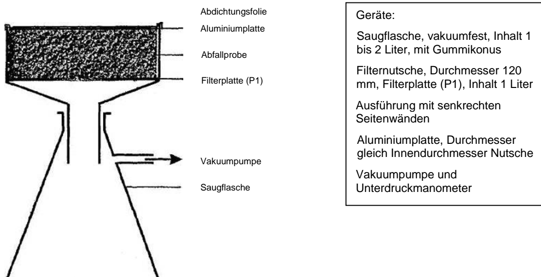
Bild 1: Apparatur zur Einstellung des Wassergehaltes
